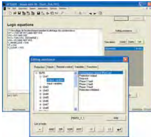
Пример экрана программного обеспечения SFT2841: редактор логических уравнений.
