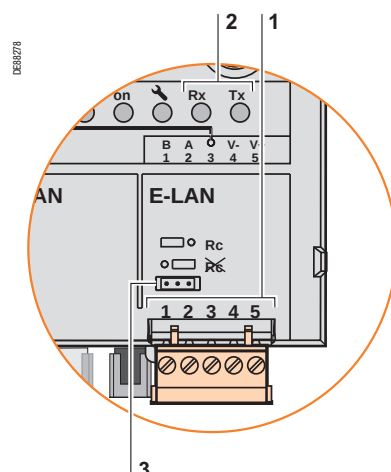
Порт E-LAN (ACE969TP или ACE969FO)
