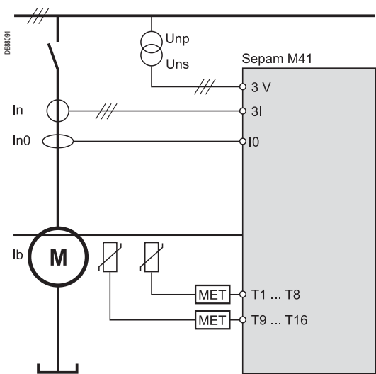
Входы датчиков Seram M41
