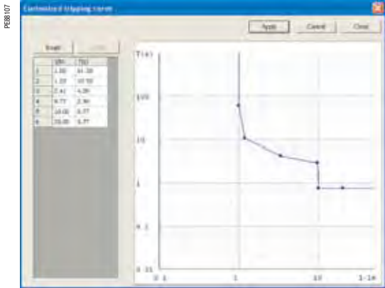
Задание персонализированной кривой отключения с помощью программного обеспечения SFT2841
