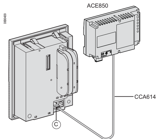
Sepam серии 40
