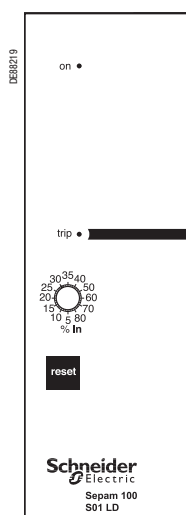
Sepam 100 LD: передняя панель
