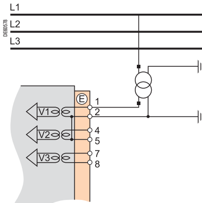
Вариант 4: измерение одного фазного напряжения (1 V)
