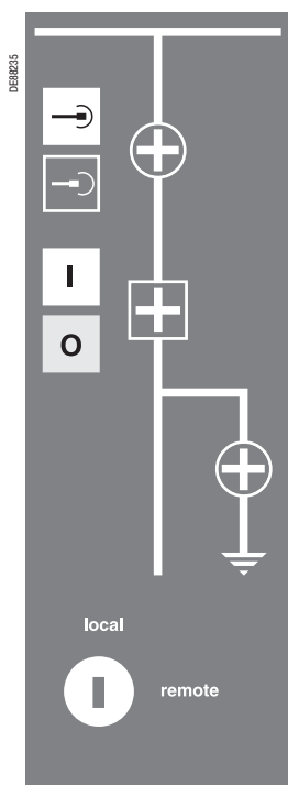
Вид спереди Sepam 100MI-X03
