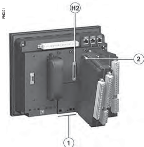
Установка второго модуля MES 120 с подключением его к разъему H2 базового блока
