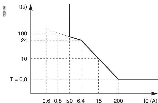
Стандартная кривая EPATRC-C (логарифмическая шкала)
