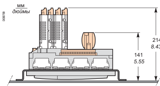
Серам с модулем MES120. Вид сверху, с монтажной платой AMT880 и пружинными зажимами
