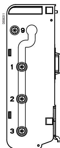
Соединение зажимов 1, 2 и 3
