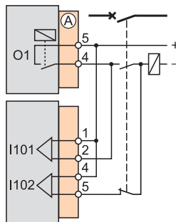
Схема присоединения для управления катушкой отключения при подаче напряжения
