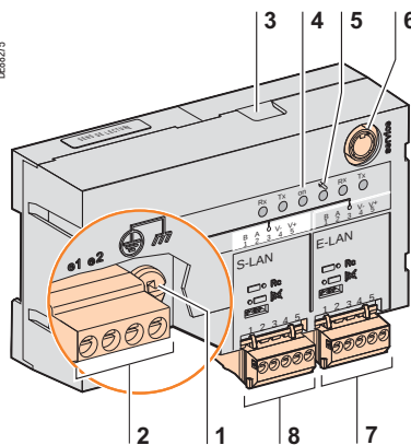
Модуль ACE969TP-2
