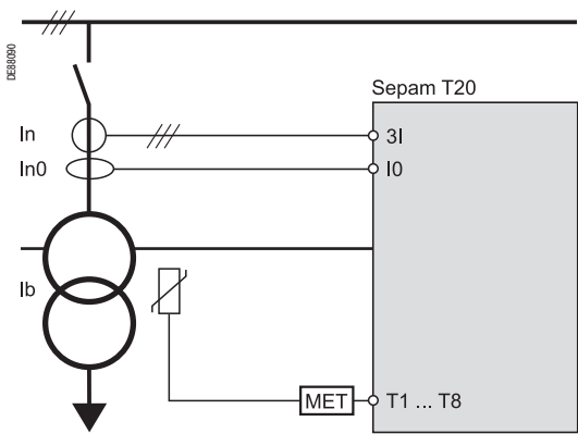
Входы датчиков Seram T20
