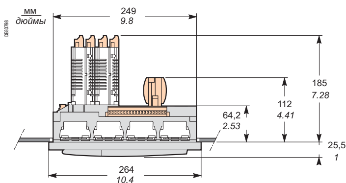
Серам с модулем MES 120. Вид сверху. Установка на передней панели ячейки заподлицо, с креплением пружинными зажимами
