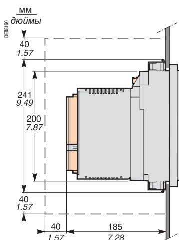
Серам с модулем MES 120. Вид сбоку. Установка на передней панели ячейки заподлицо, с креплением пружинными зажимами.
