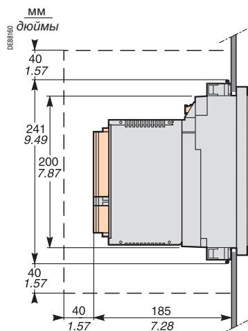
Серам с модулем MES 120. Вид сбоку. Установка на передней панели ячейки заподлицо, с креплением пружинными зажимами. Толщина передней панели ячейки: 1,5 - 6 мм
