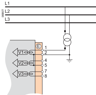
Вариант 3: измерение одного линейного напряжения (1 U)
