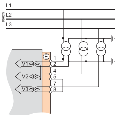
Вариант 1: измерение трех фазных напряжений (3 V, стандартная схема подключения)
