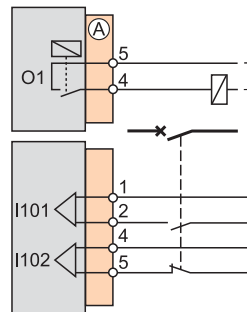
Схема присоединения для управления катушкой отключения при исчезновении напряжения
