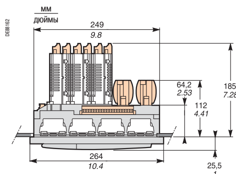
Серам с модулем MES 120. Вид сверху. Установка на передней панели ячейки заподлицо, с креплением пружинными зажимами. Толщина передней панели ячейки: 1,5 - 6 мм
