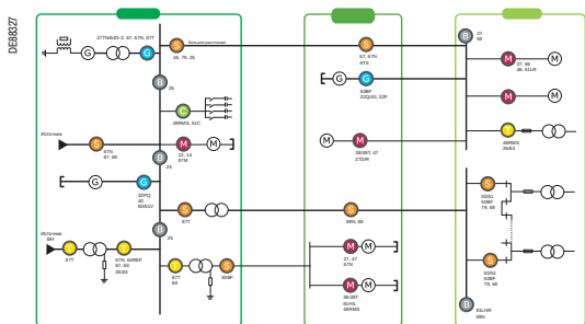
ABP с контролем синхронизма с Серам серии 80
