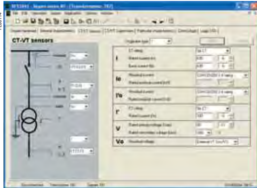
Пример экрана программного обеспечения SFT2841: настройка параметров датчиков Sepam серии 80
