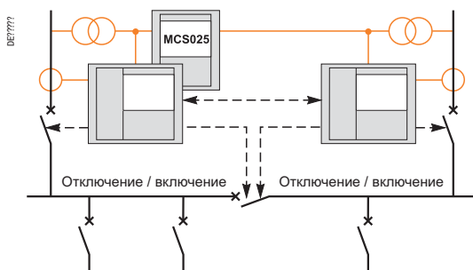
ABP с контролем синхронизма с Серам серии 60
