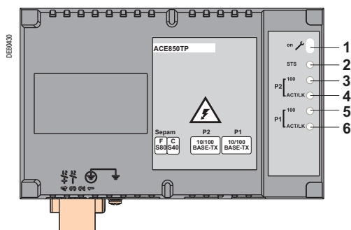
Модуль ACE850TP: вид спереди
