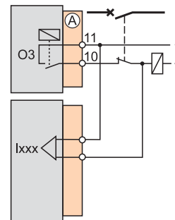
Схема присоединения для управления цепью включения
