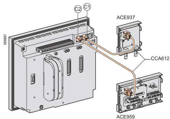
Sepam серии 80: 2 порта связи
