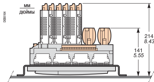
Серам с модулем MES120. Вид сверху, с монтажной платой AMT880 и пружинными зажимами. Монтажная плата: толщина 3 мм.
