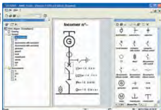
Пример экрана программного обеспечения SFT2841: редактор мнемосхемы
