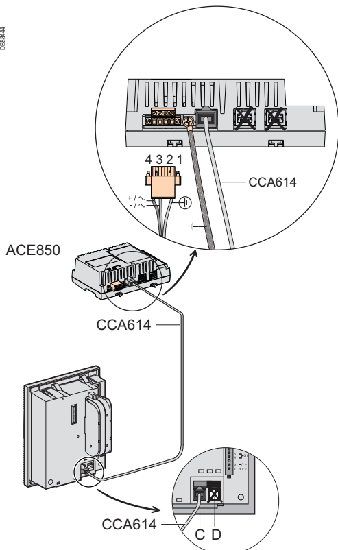
Подключение модуля ACE850 к устройству Seram серии 40
