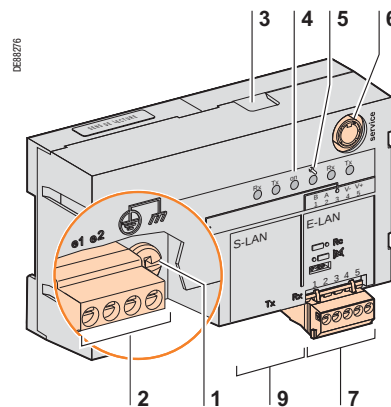
Модуль ACE969FO-2
