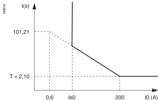
Стандартная кривая EPATRB-C (логарифмическая шкала)
