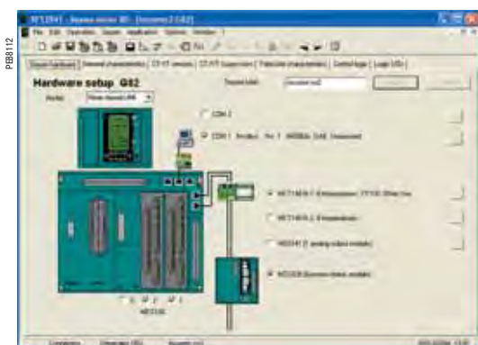
Пример экрана программного обеспечения SFT2841: аппаратная конфигурация Sepam серии 80
