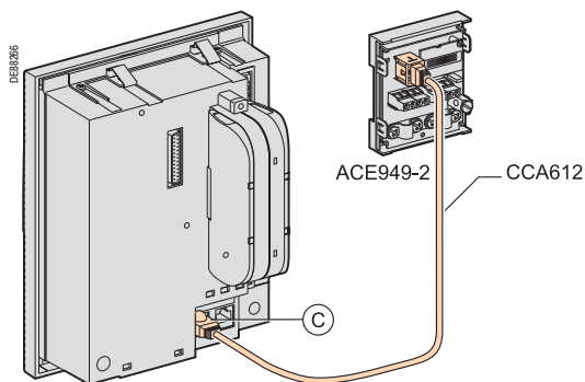
Sepam серий 20 и 40: 1 порт связи
