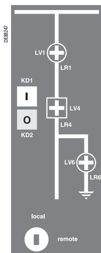
Мнемосхема Serap 100MI-X02
