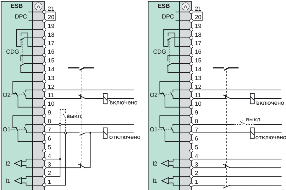
Плата ESB
