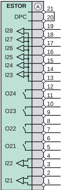
Плата ESTOR2 для типов B02, B04, S07, S08
