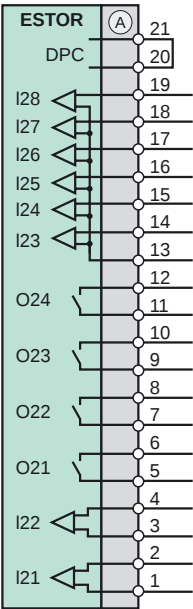
Плата ESTOR2 для типа B07
