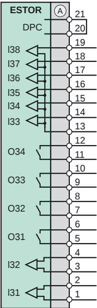
Carte ESTOR3 type B07
