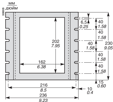
Монтажная панель AMT840
