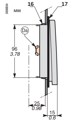
Вид сбоку
