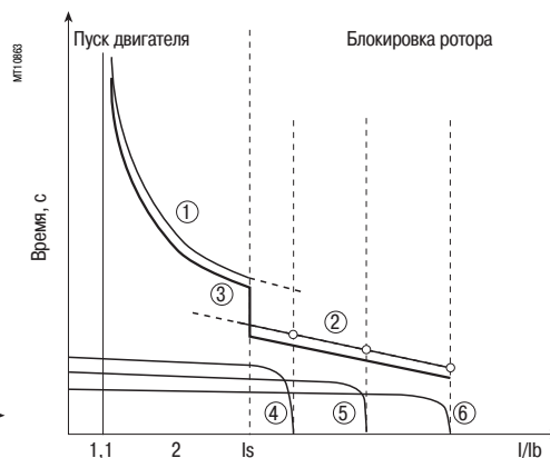
Рисунок 4: тепловые характеристики заблокированного ротора
