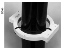
Монтаж на кабелях среднего напряжения
