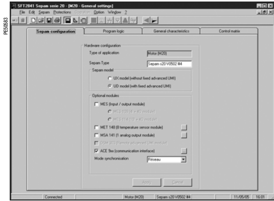
SFT2841: Экран конфигурации Sepam
