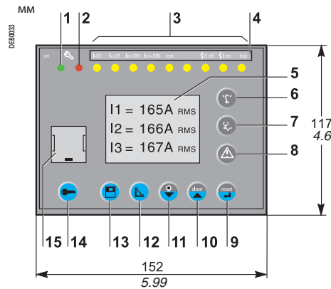
Вид спереди
