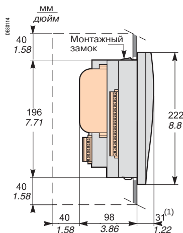
Sepam с усовершенствованным UMI и MES114, утолщенный монтаж на передней панели
