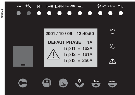
Аварийные сообщения на дисплее усовершенствованного UMI
