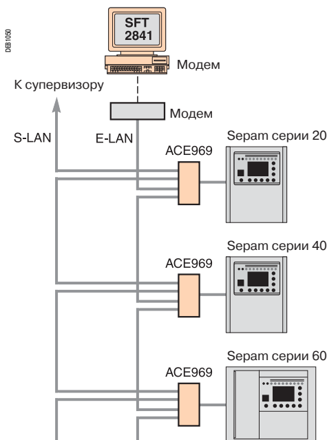
Система SFT2841, подключенная к сети Sepam
