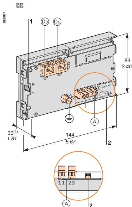
(1) 70 мм с присоединенным кабелем CSA 77x
