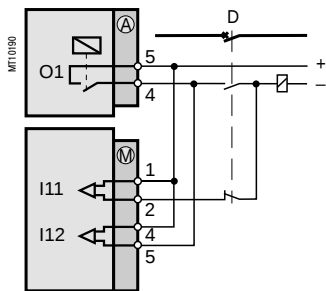
Схема для блока расцепления через реле параллельно включенной катушке
