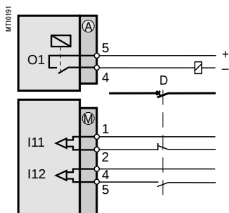
Схема для устройства расцепления минимального напряжения
