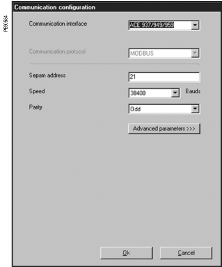
SFT2841: окно конфигурации связи для ACE949
