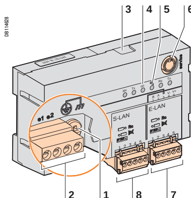
Модуль ACE 969TP-2
