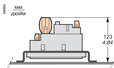
Sepam со стандартными UMI и MES114, установленный на панели AMT840 Толщина монтажной панели: 2 мм (0,079 дюйма).
