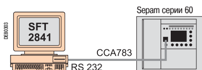
Система SFT2841, подключенная к одному устройству Sepam с последовательным портом
