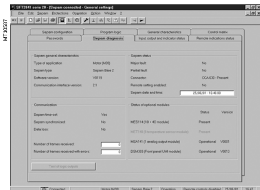
Пример экрана «Диагностика Sepam» программного обеспечения SFT 2841
