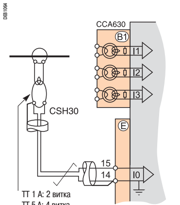
Подключение к промежуточному кольцевому тору CSH 30
