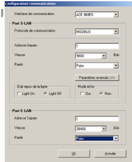
SFT2841: окно конфигурации связи для ACE969FO
